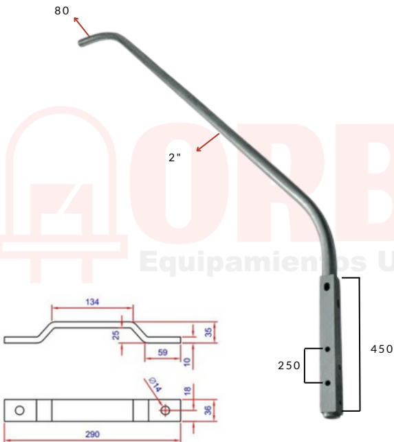
Detalle abrazadera
