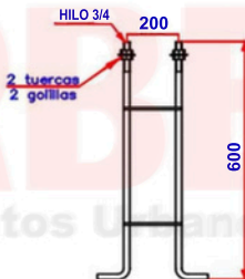
DETALLE PLACA BASE
