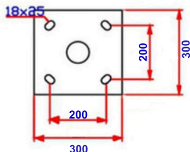
DETALLE PLACA BASE
